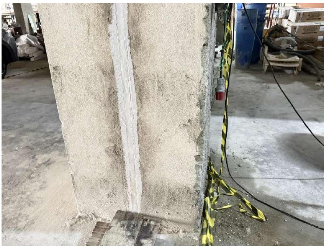
Figura 28 Instalação de junta de movimentação nos pilares do pavimento semienterrado 2.
